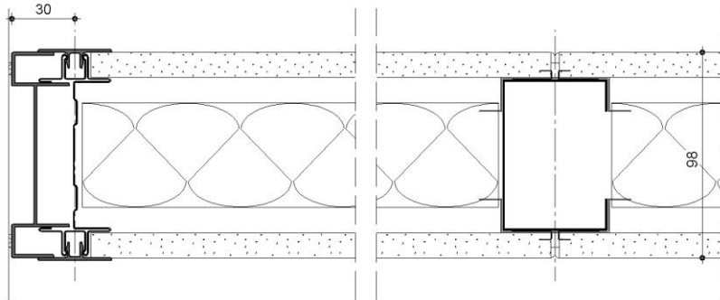
Wandanschluss M 1:2
